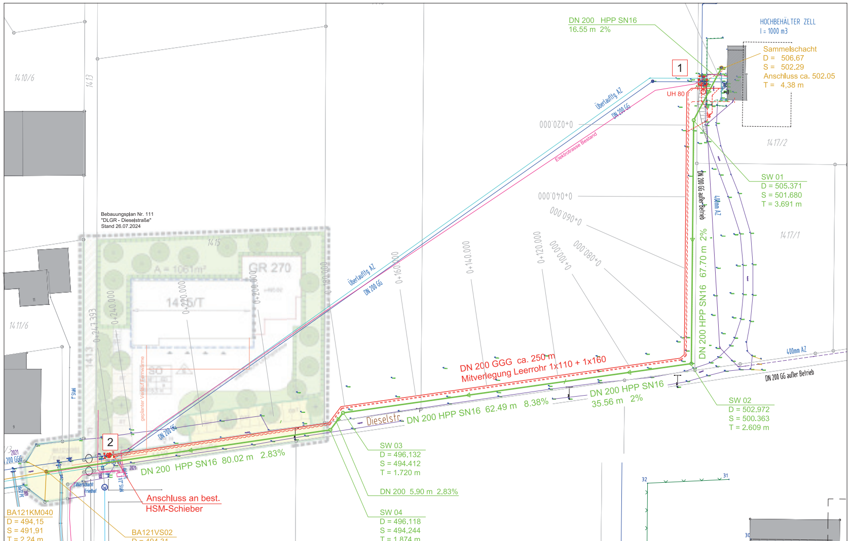
TW-Hochbehälter Zell, Neubau Überlaufleitung, Ausführungslageplan
